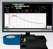
ECNI-II
