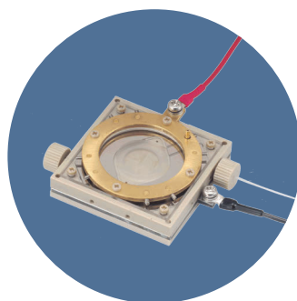
超小型電解セル 電解液を流しながら通電し、 反応面（析出面）を上部から観察できる 超小型めっき槽です 液量約 30 \mu L
